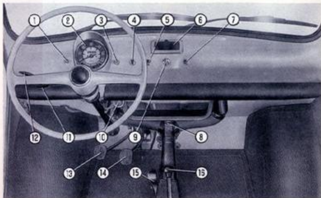
Vettura con guida a sinistra.
