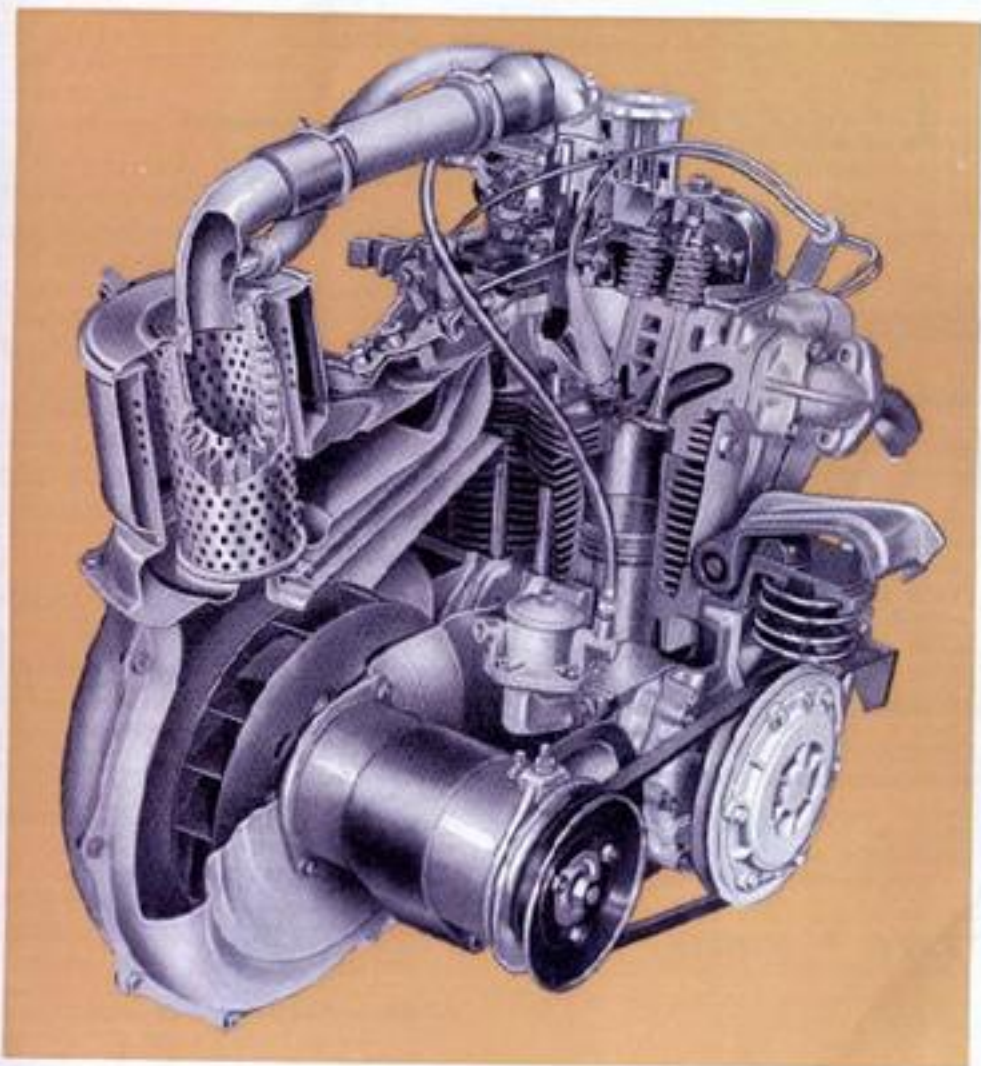
Motore con ventilatore, sezionati parzialmente
