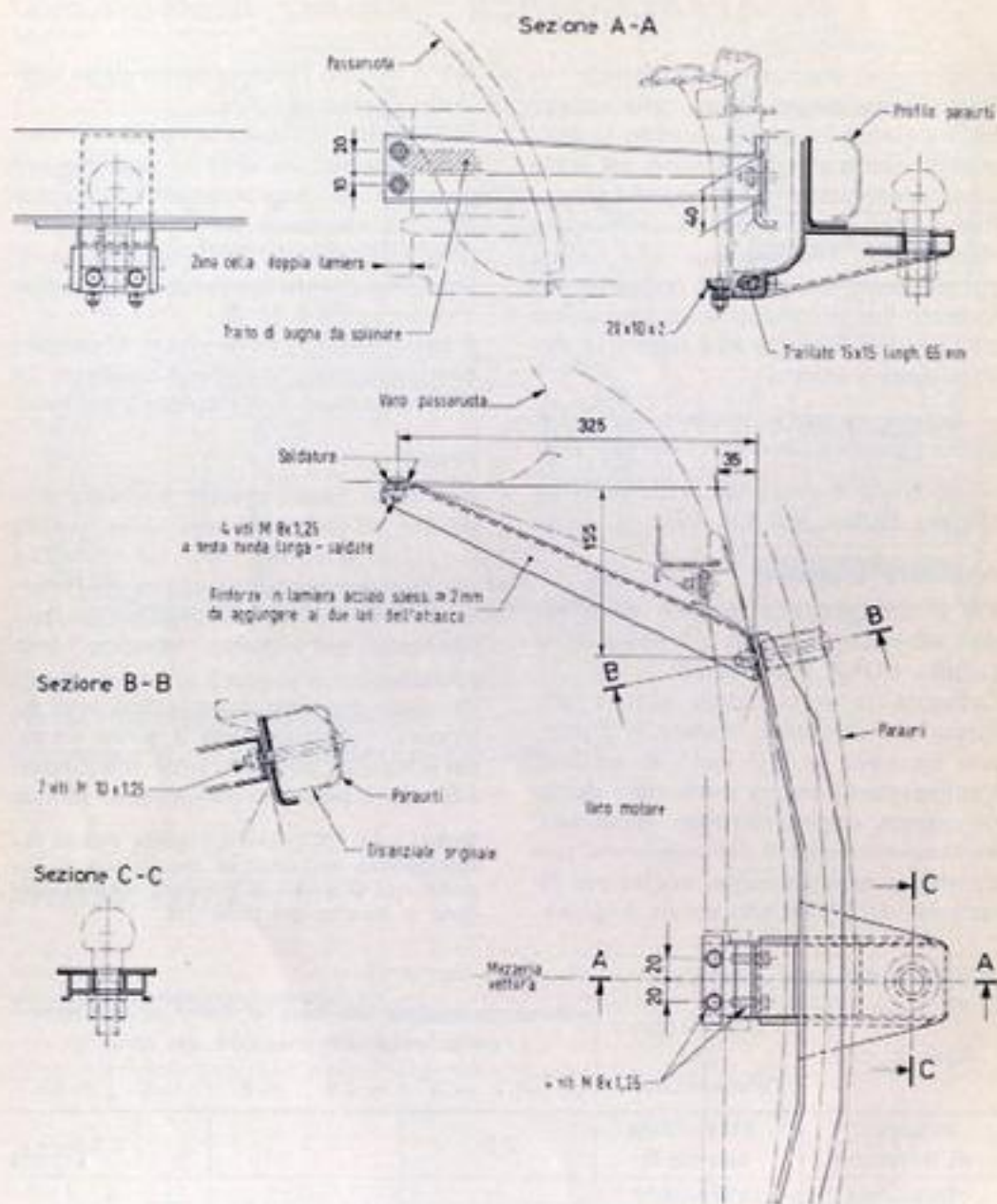
Installazione attacco traino rimorchio
